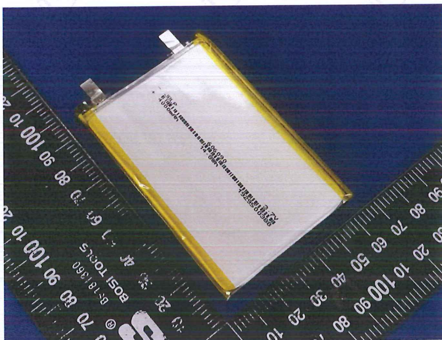
606090图1 电池（正面）
